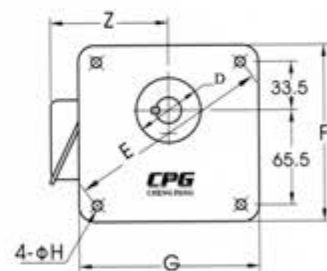
B 型法蘭 B TYPE FLANGE
